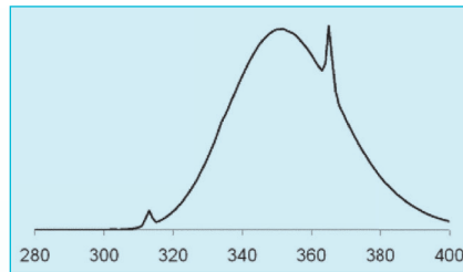
UVA
