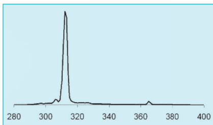
UVB-311
